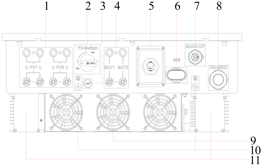
图 4.1 逆变器外观图
